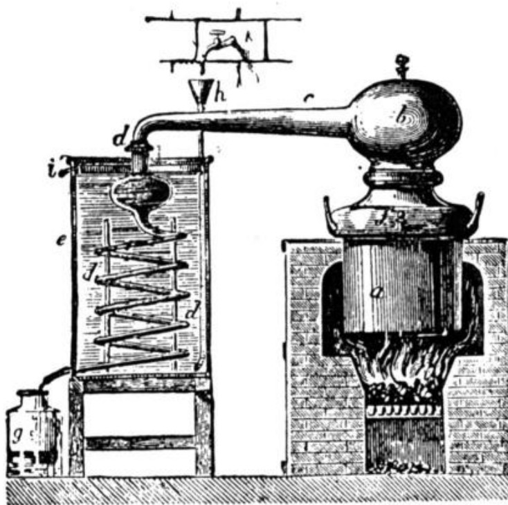
Рис. 15. Перегонный кубъ.
