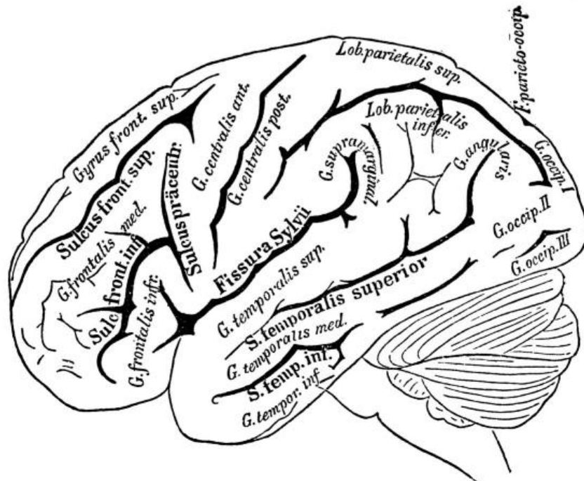
Рис. 2. Борозды и извилины поверхности лѣваго полушарія Gyrus означаетъ извилина; Lob (lobus)—доля; fissura—борозда; sulcus—борозда; Fissura Sylvii—Сильвиева борозда; G. frontalis—лобная извилина; sup.—верхняя; med.—средняя; inf.—нижняя; G. centralis—центральная извилина. ant.—передняя; post.—задняя; G. occip.—затылочная извилина; G. temporalis—височная извилина.
